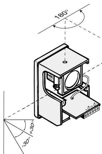
OTTICA ORIENTABILE
