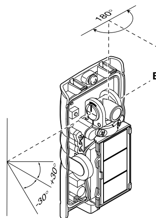
OTTICA ORIENTABILE
