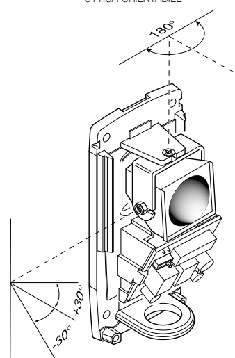
OTTICA ORIENTABILE
