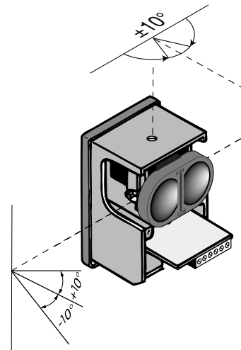
OTTICA ORIENTABILE
