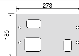
BASE DI FISSAGGIO CODICE DI RICAMBIO 999805
