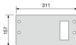
BASE DI FISSAGGIO CODICE DI RICAMBIO 999393
