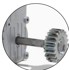
PIGNONE ESTRAIBILE
