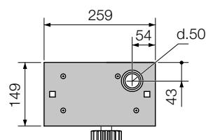
BASE DI FISSAGGIO CODICE DI RICAMBIO 9992026
