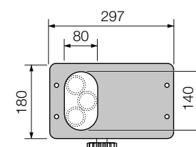
BASE DI FISSAGGIO CODICE DI RICAMBIO 9995114
